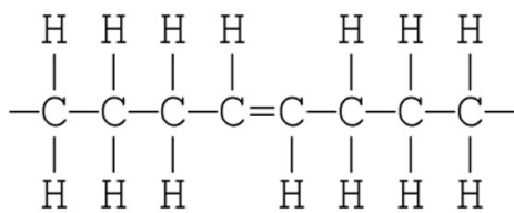
Abb. 5: trans-Konfiguration. Urgeschmack, 12.09.2012.
